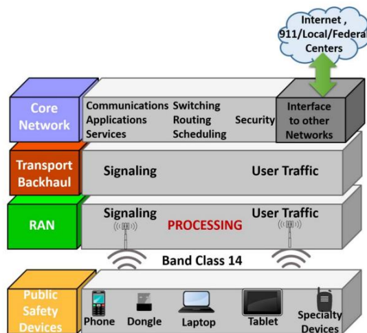
Εικόνα 108. Αρχιτεκτονική LTE για το FirstNet [148]
