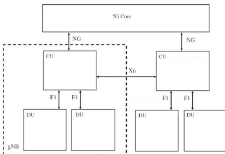
Εικόνα 32. NG-RAN κεντροποιημένο και κατακευματισμένο σύστημα [77]
