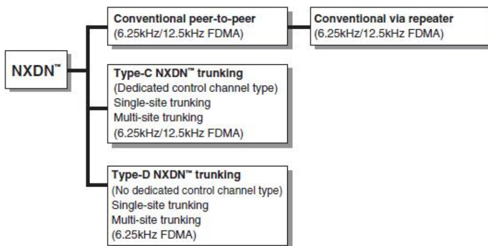
Εικόνα 98. Πρότυπο NXDN [267]
