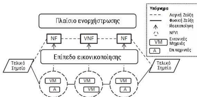
Εικόνα 29. NVF πλαίσιο [75]
