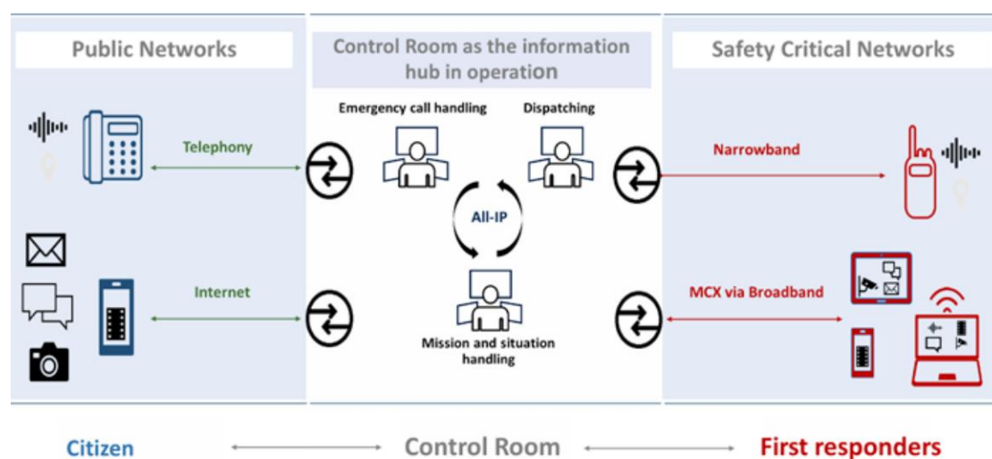
Εικόνα 159. Μοντέλο επικοινωνιών πολιτών και πρώτων ανταποκριτών με το κέντρο ελέγχου και διοίκησης [410]
