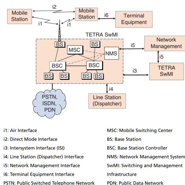
Εικόνα 90. Αρχιτεκτονική του δικτύου TETRA [59]
