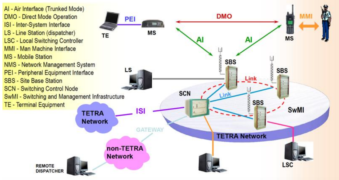
Εικόνα 91. Κύρια στοιχεία και διεπαφές δικτύου TETRA [252]
