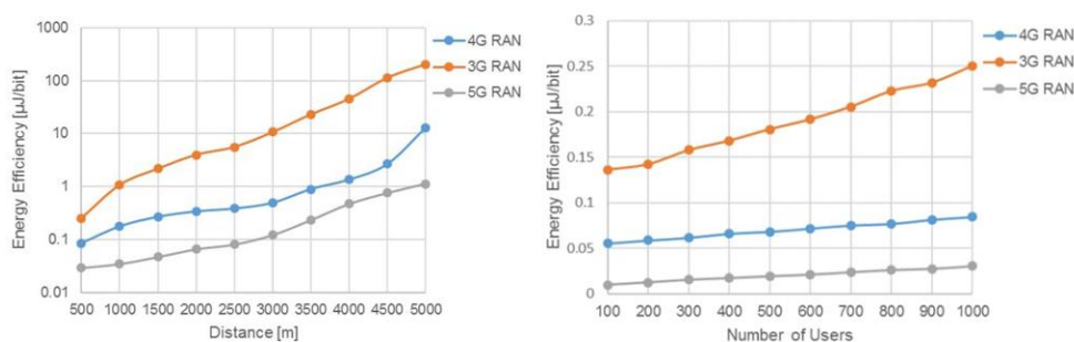
Εικόνα 35. Ενεργειακή απόδοση ως συνάρτηση της (α) απόστασης μεταξύ κάθε RAN και της έξυπνης συσκευής του χρήστη και (β) αριθμό έξυπνων συσκευών [80]
